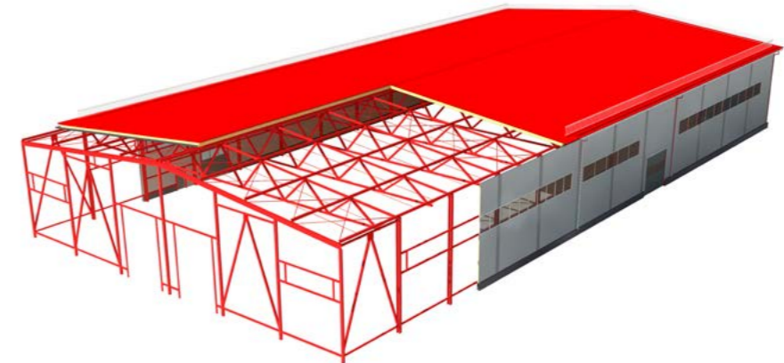
здание на основе сварной металлической фермы
